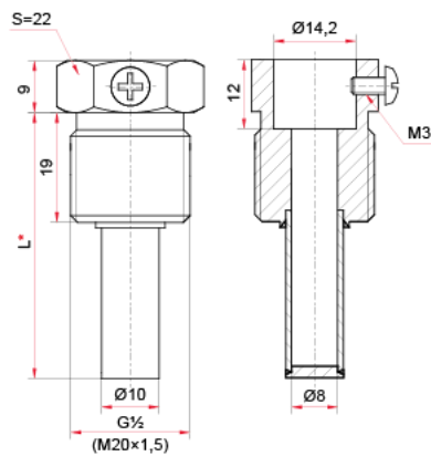
Гильза для термометров БТ серии 211
