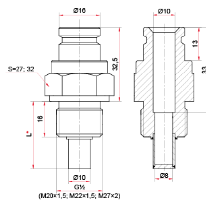
Гильза для термометров ТТ-В (РЧ Исп. 2 – угловые)
