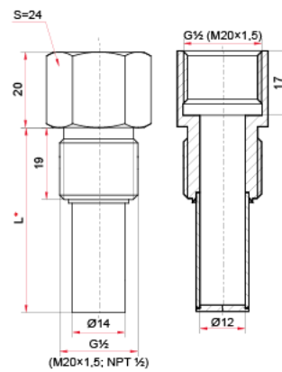
Гильза для термометров БТ серии 220
